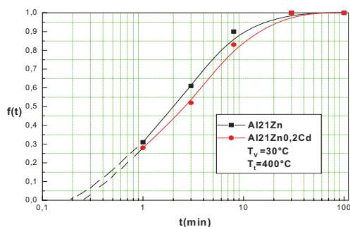
Figure 3. Cinétique de précipitation des zones GP dans Al-Zn et Al-Zn-Cd
