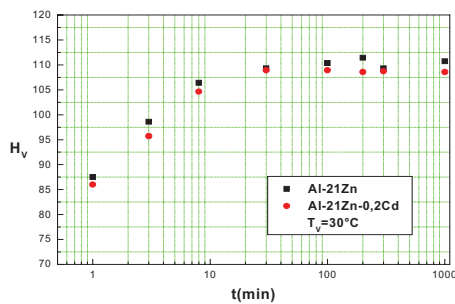
Figure 2. Isothermes de dureté de Al-Zn et Al-Zn-Cd
